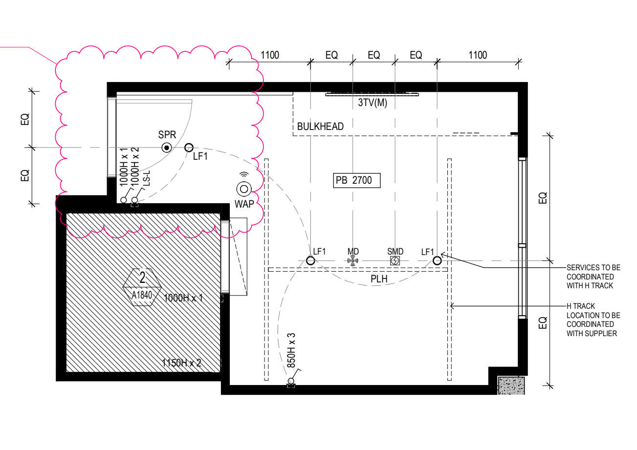
2 RCP-STANDARD BEDROOM - TYPE A Scale 1 : 50
